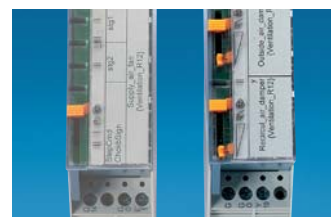
DESIGO I/O modulok kézi vezérléssel és felirattal
