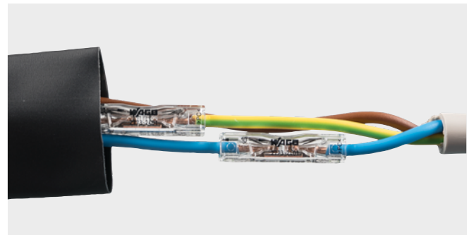
Alkalmazás zsugorcsonnyal
