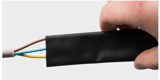
Helyezze fel a zsugorcsővet.
