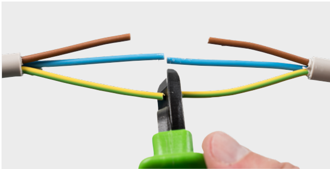
Vágja el, majd csupaszolja a kábelt és a vezetékeket.
